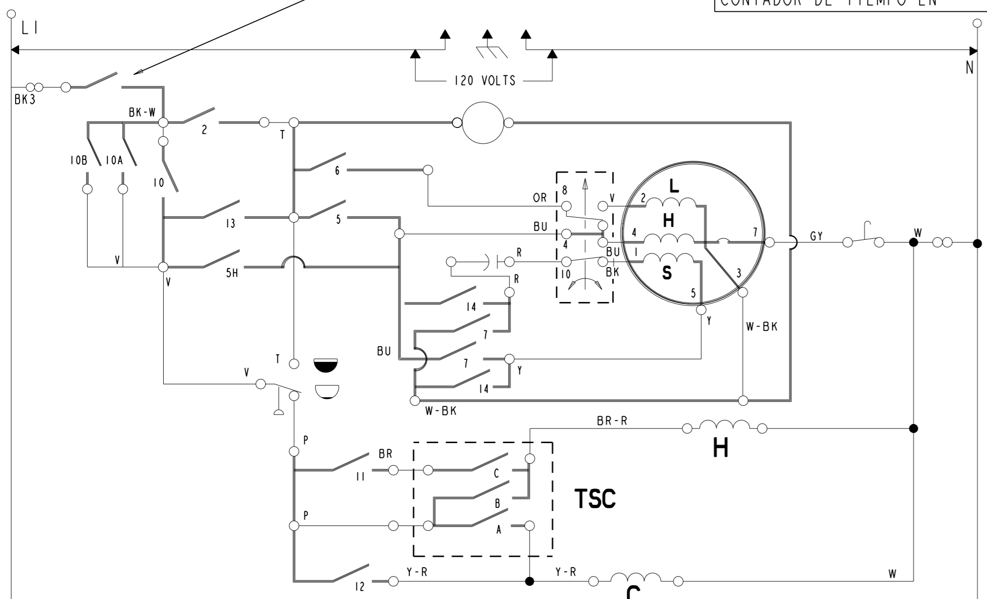
WASHER WIRING DIAGRAM / DIAGRAMME DE CABLAGE DE RONDELLE / DIGRAMA ELECTRICO DE LA ARANDELA
