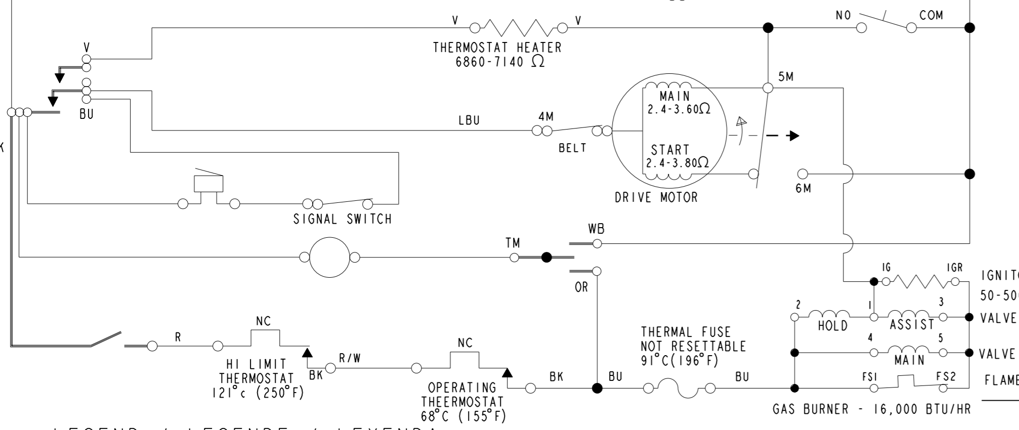
DRYER WIRING DIAGRAM / DIAGRAMME DE CABLAGE DE DESSICCATELLR / DIGRAMA ELECTRICO DEL SECADOR
