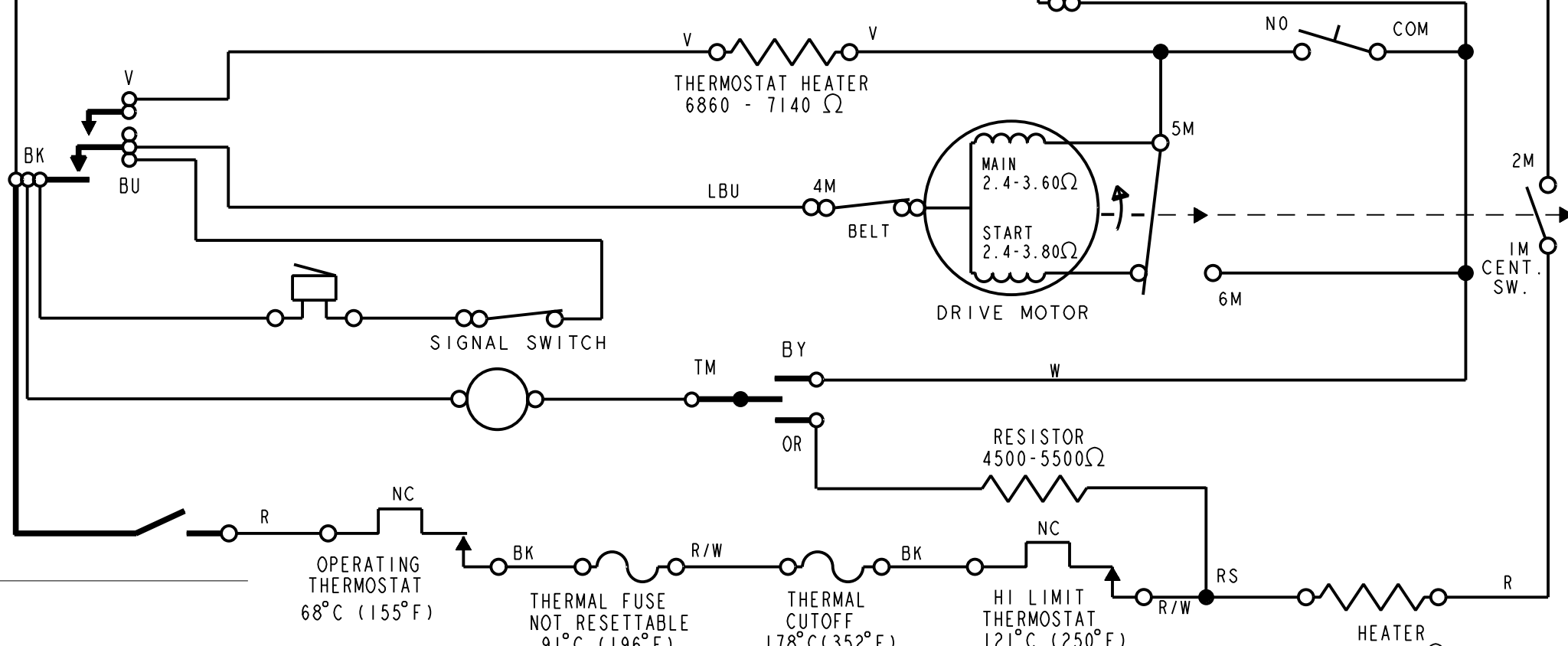
DRYER WIRING DIAGRAM / DIAGRAMME DE CABLAGE DE DESSICCATELLR / DIGRAMA ELECTRICO DEL SECADOR
